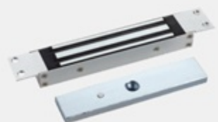
ZU-280A、ZU-280AF (280KG 暗装两线/反馈磁力锁)
